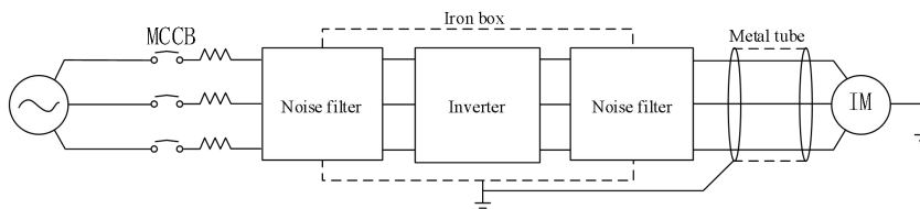
Рис.3-9 Решение проблемы радиочастотных помех
