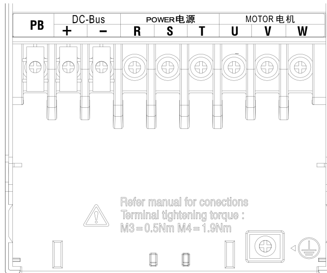
b) EM730-5R5-3В~EM730-022-3В
