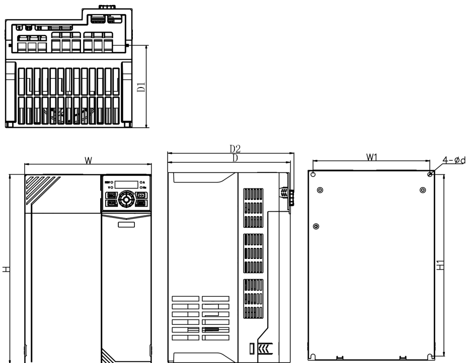
(a) Размеры моделей от EM730-0R7-3B до EM730-022-3B
