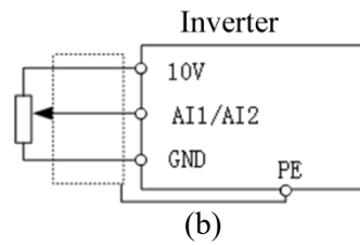
Рис.3-12 схема подключения к клеммам AI1/AI2
