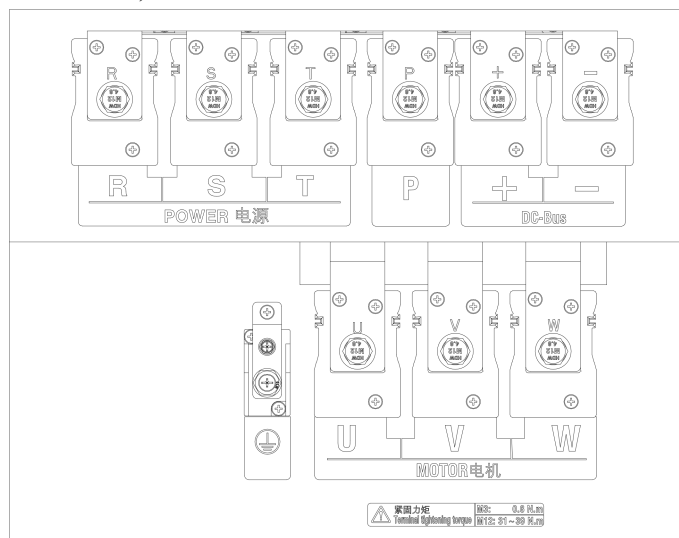
f) EM730-132-3~EM730-160-3
