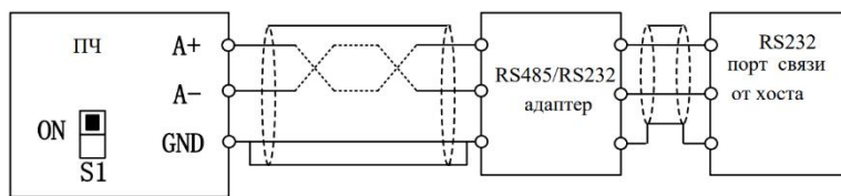
Рис. 3-18 Подключение к клеммам
