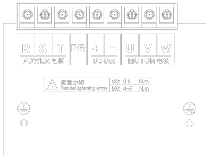
b) EM730-5R5-3В~EM730-022-3В
