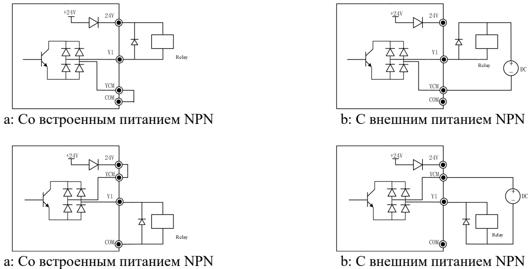
Рис.3-15 Подключение к выходным клеммам управления
