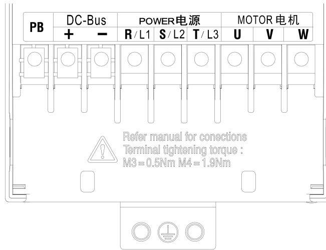
b) EM730-2R2-3В~EM730-4R0-3В
