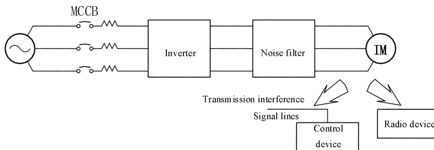
Рис.3 7 Установка фильтра помех на выходной стороне
