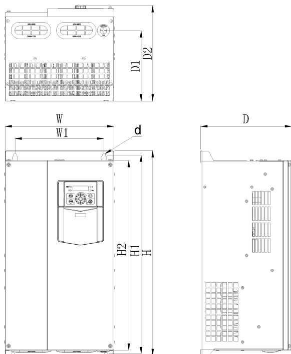
(b) Размеры моделей от EM730-030-3B до EM730-075-3
