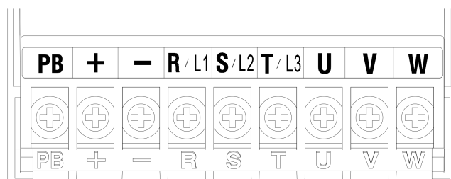
а) EM730-0R7-3B~EM730-1R5-3B
